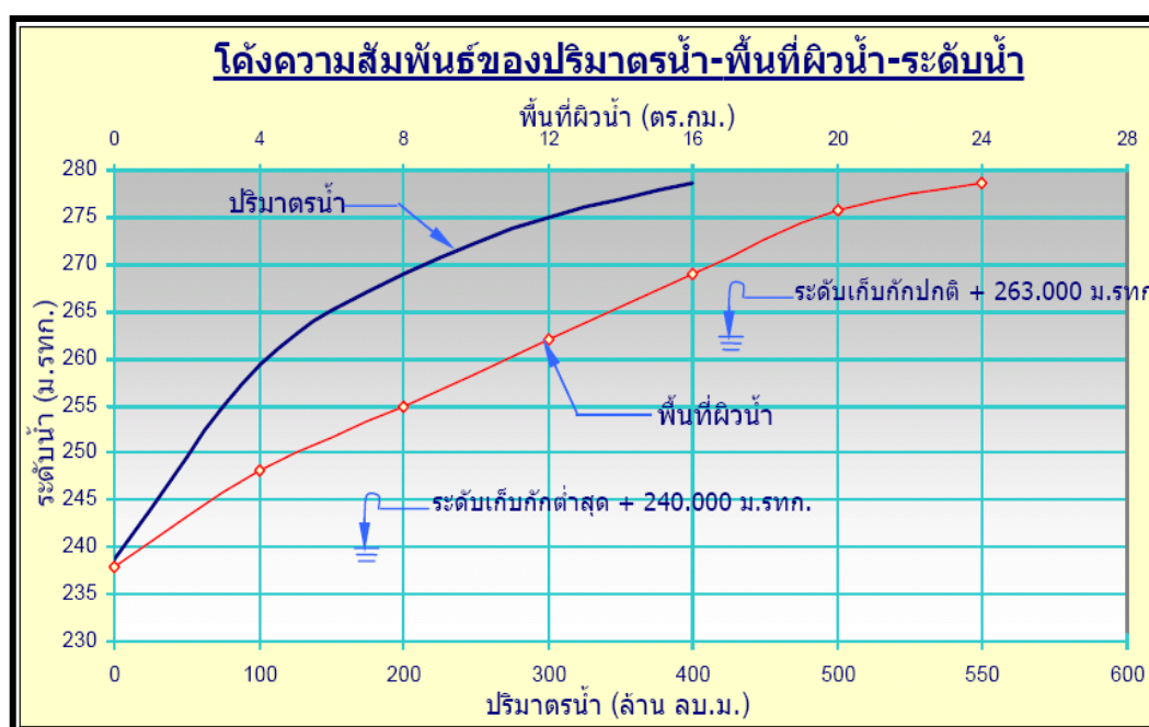
รูปที่ 2.5 โค้งความสัมพันธ์ของปริมาณน้ำ-พื้นที่ผิวน้ำ-ระดับน้ำ
