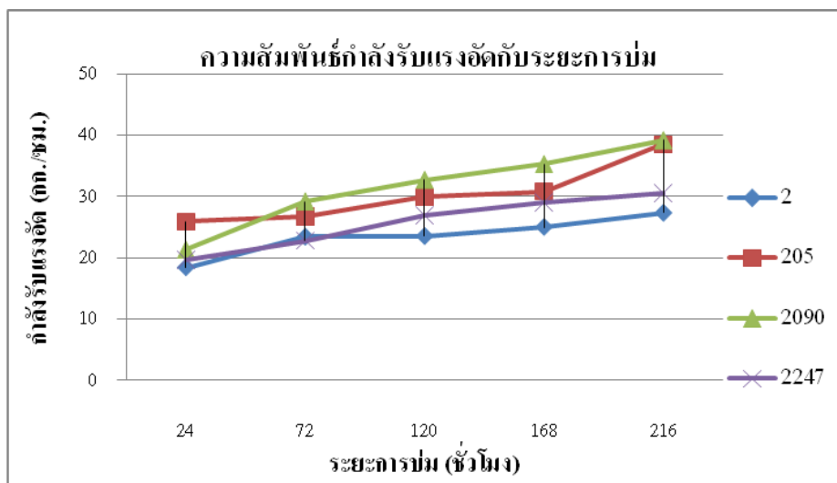
รูปที่ 4.17 กราฟแสดงกำลังรับแรงอัดเฉลี่ยตามระยะการบ่มของ 4 สายทาง
