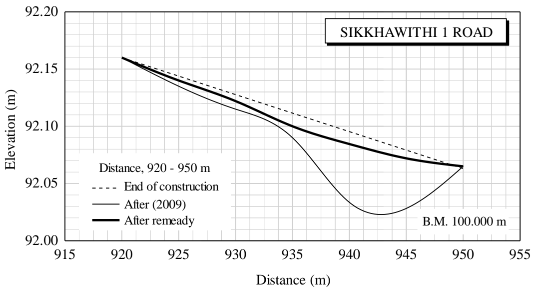
รูปที่ 4.20 ค่าระดับถนนสิกขวิที 1 (SKR1.1, SKR1.2) หลังปรับปรุง
