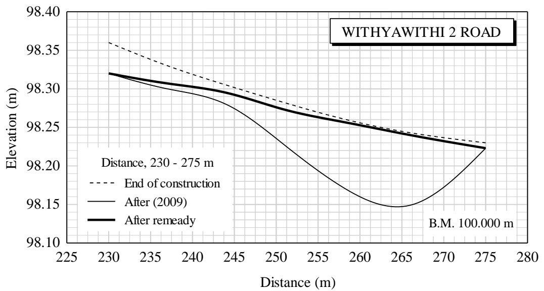
รูปที่ 4.22 ค่าระดับถนนวิถยวิถึ 2 (WTR2) หลังปรับปรุง
