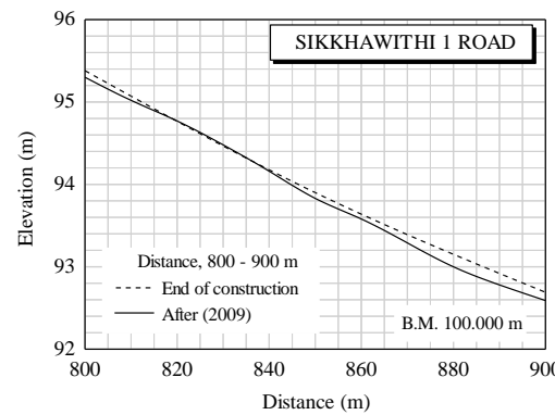
รูปที่ 4.1 ค่าระดับถนนวิฑยวธิ 1 ถึง ถนนสิขหวธิ 1
