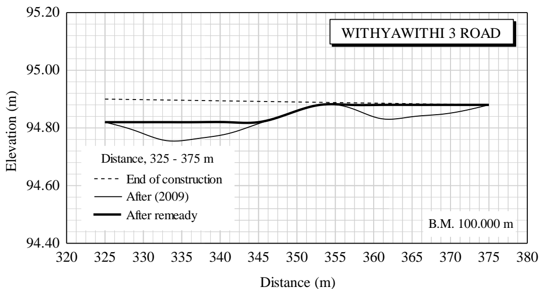
รูปที่ 4.23 ค่าระดับถนนวิทย์วิถี 3 (WTR3) หลังปรับปรุง
