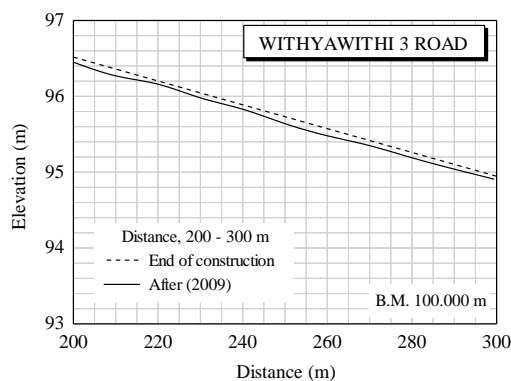
รูปที่ 4.5 ค่าระดับถนนวิทวีถิ 3
