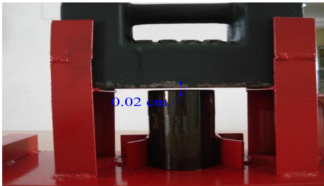
ภาพการวางกระบอกลมผสมวัสดุเข้ากับชุดทดลอง
