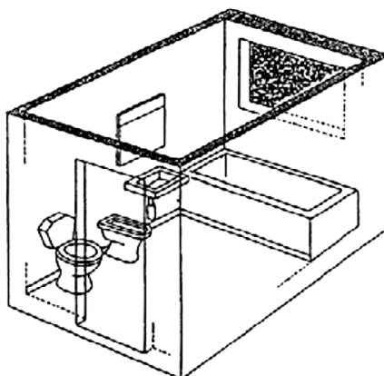
รูปที่ 2.19 ห้องน้ำคอนกรีตสำเร็จรูป
